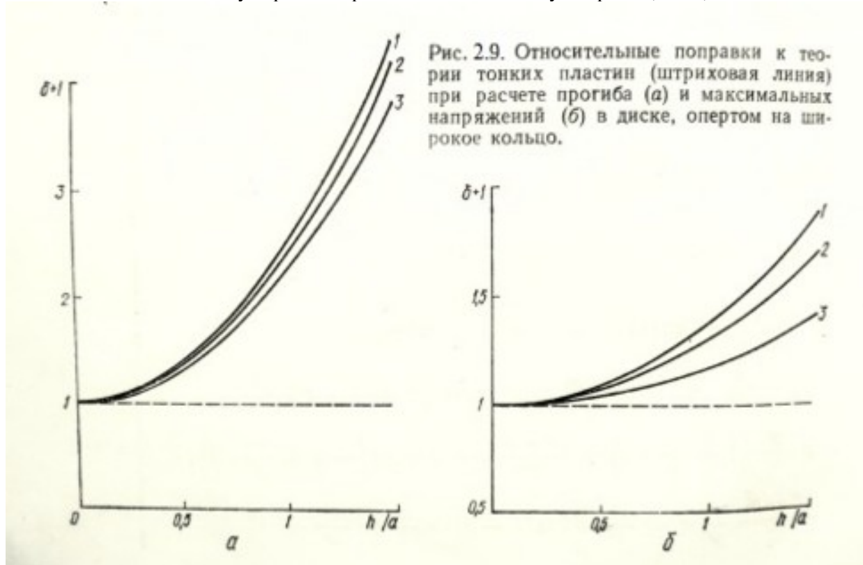
Рисунок 2.9. Относительные поправки к теории тонких пластин (штриховая линия с единичной ординатой) при расчёте стрелы прогиба (а) и максимальных напряжений (б) именно существенно трёхмерного сплошного цилиндрического тела, в частности светопрозрачного элемента, при изгибе равномерным давлением на одно основание и равномерным противодействием на периферическую часть другого основания со свободной центральной частью.
