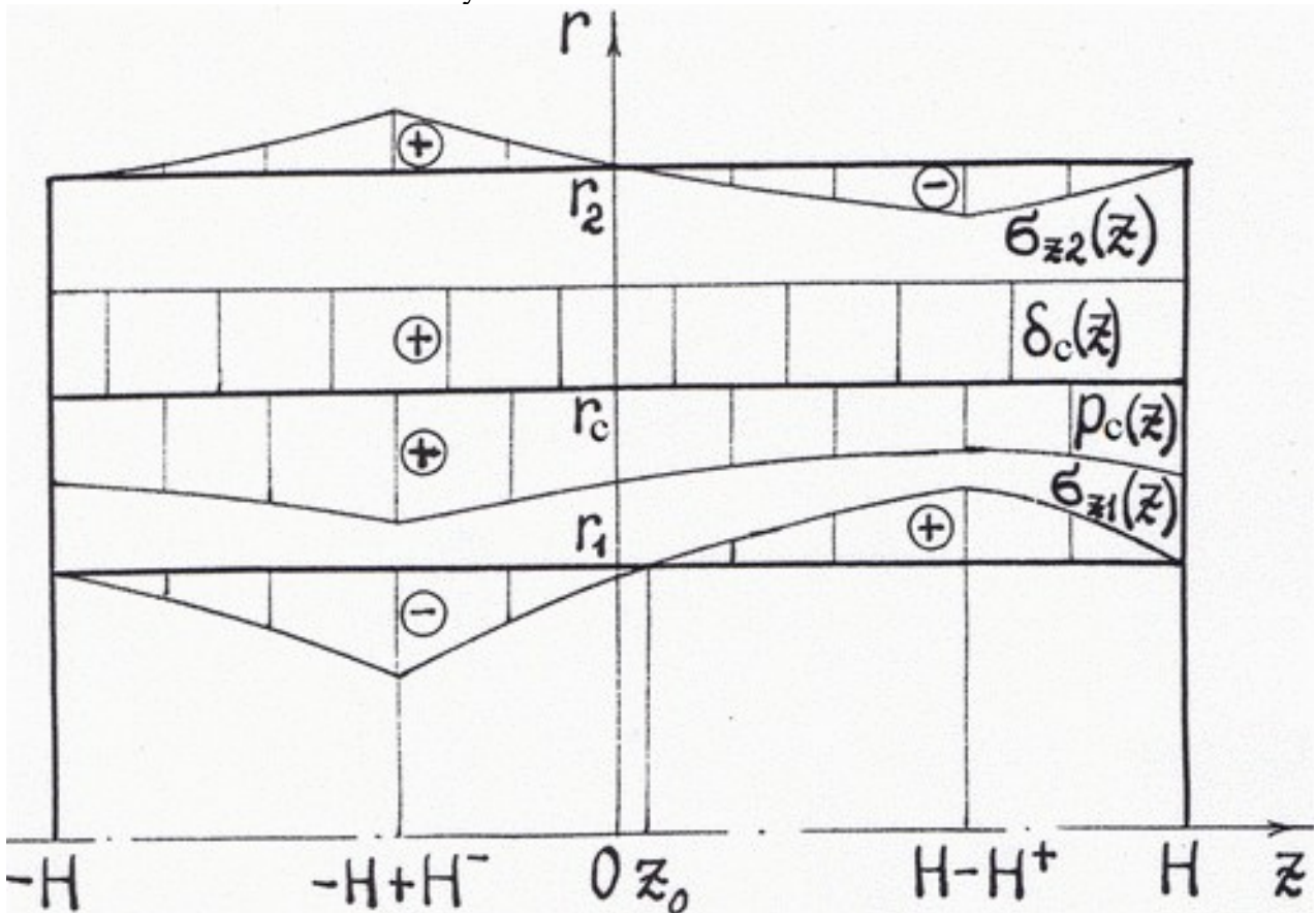
Рисунок 5.3. Эпюры относительного натяга \delta_c(z) и сборочных контактного давления \rho_c(z) и осевых напряжений \sigma_{z1}(z) и \sigma_{z2}(z) в слоях собранного запрессовкой составного цилиндра конечной длины с равномерным вдоль оси натягом после сброса усилия запрессовки в установившемся состоянии.
