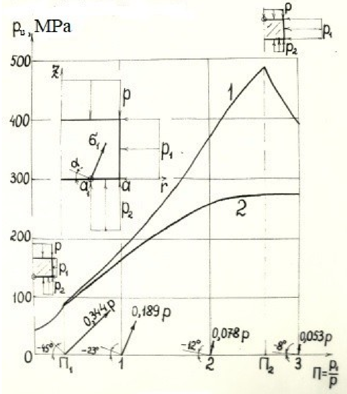
Рисунок 3.1. Влияние относительной (к внешнему давлению p ) величины \Pi = r_1/p давления p_1 , приложенного к боковой поверхности нагруженного по схеме основного типа в технике высоких давлений (с повышенным периферическим противодействием) именно существенно трёхмерного сплошного цилиндрического тела, в частности светопрозрачного элемента, из неорганического стекла К8 с соотношением размеров h:a_1:a = 2:1:(11/6) , на величину и ориентацию разрушающего главного напряжения \sigma_1 и на вероятный угол \alpha скалывания далее растрескиваемого сегмента у края ненагруженной центральной части частично нагруженного основания, на положение (кружок в центре или на краю центральной части частично нагруженного основания) места наибольшего равносильного (эквивалентного) напряжения в теле (светопрозрачном элементе) и на давление его разрушения p_u по первой теории прочности (и приведённой) и приведённому критерию Г. С. Писаренко и А. А. Лебедева (кривая 1), по критериям Г. С. Писаренко и А. А. Лебедева, Кулона–Мора, приведённой третьей теории прочности и приведённой четвёртой теории прочности (кривая 2).
